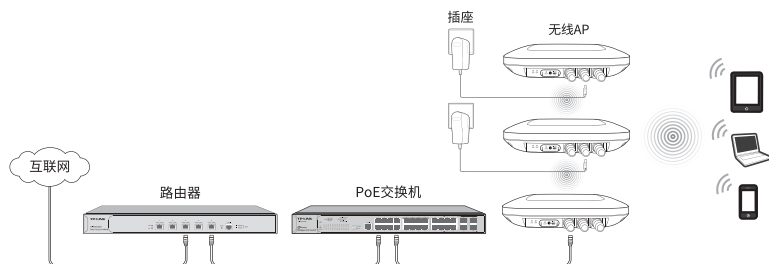
图4-2 典型应用拓扑图-易展分布式无线组网（一）
